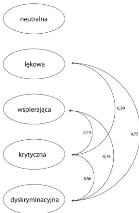
Rysunek 7. Korelacje pomiędzy poszczególnymi skalami.
