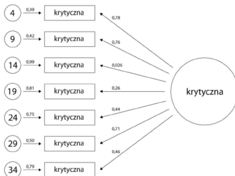
Rysunek 5. Wyniki konfirmacyjnej analizy czynnikowej pozycji przynależących do skali krytycznej.
