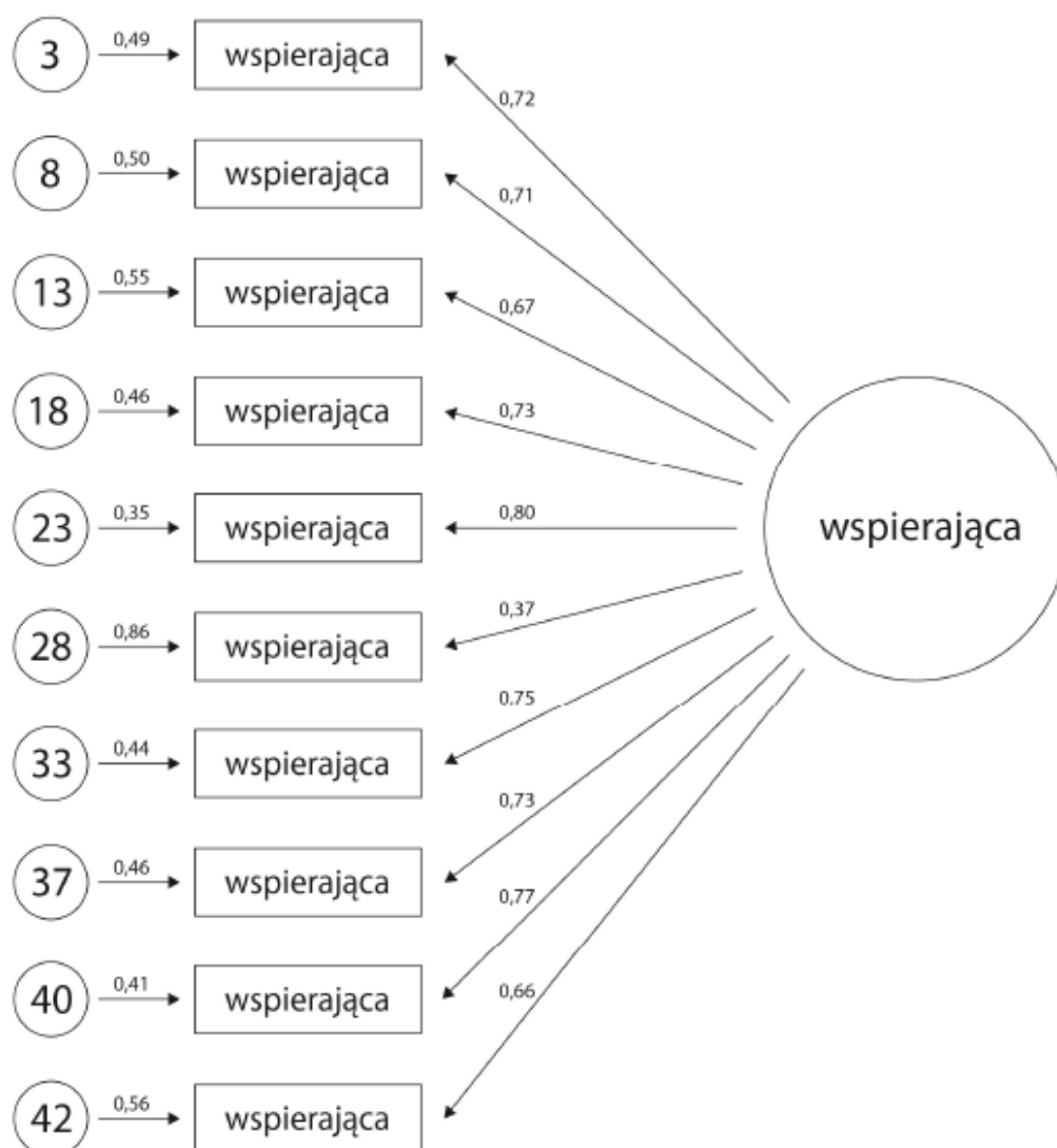
Rysunek 6. Wyniki konfirmacyjnej analizy czynnikowej pozycji przynależących do skali wspierającej.
