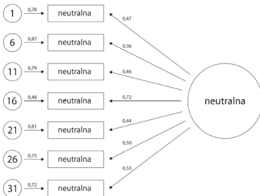
Rysunek 2. Wyniki konfirmacyjnej analizy czynnikowej pozycji przynależących do skali neutralnej.
